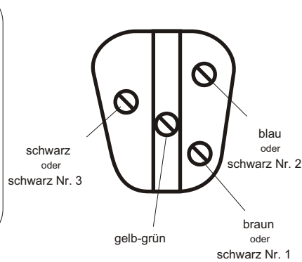
Belegung Zwischenstecker
